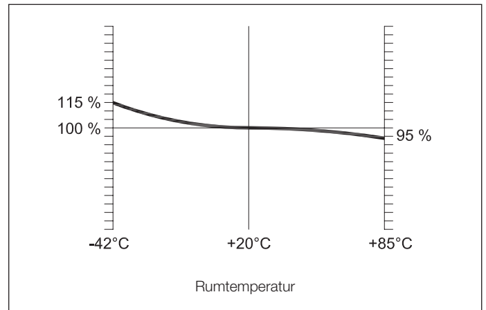
Temperatur indflydelse på reaktionskraft (N/m)
